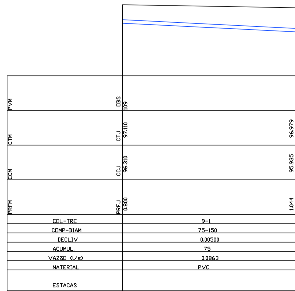
2 PERFIL DO COLETOR 9 ESCALA 1:1
