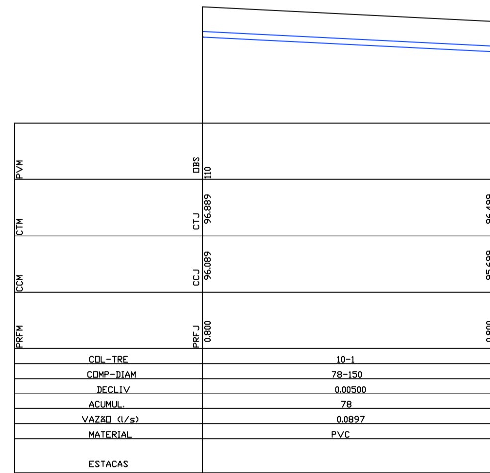
3 PERFIL DO COLETOR 10 ESCALA 1:1
